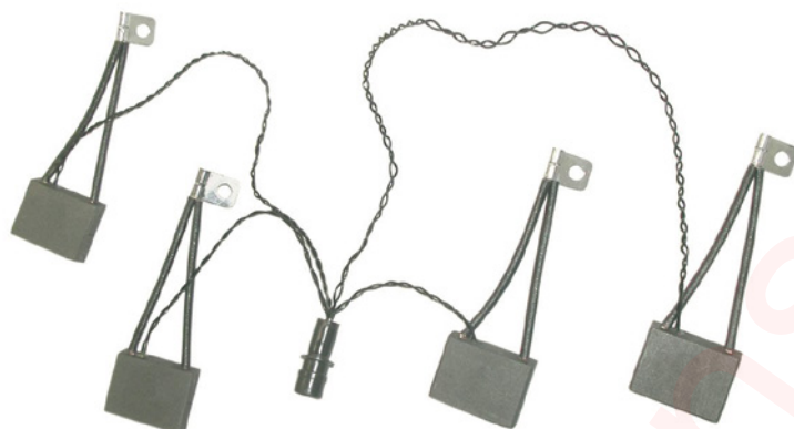
Type M4 4 balais unis
